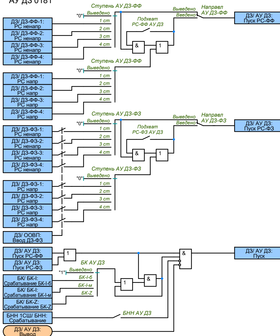
2.2.9.3 Ввод в работу пуска АУ ДЗ-ФФ(ФЗ) и выбор ускоряемой ступени задается программным переключателем «АУ ДЗ-ФФ(ФЗ)» . Предусмотрена возможность вывода направленности ускоряемой ступени с помощью программного ключа «Направл АУ ДЗ-ФФ(ФЗ)» . Контроль ускорения от блокировки при качаниях (БК) задается программным переключателем «БК АУ ДЗ» , а блокировка от БНН вводится с помощью программного ключа «БНН АУ ДЗ» . Также предусмотрена возможность подхвата направленного пуска РС от ненаправленного, задается с помощью программных переключателей «Подхват РС-ФФ(ФЗ) АУ ДЗ» .
